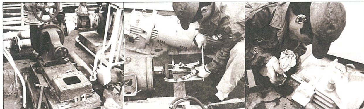
1. 旧モータ取外し 2. モータ側旧カップリング抜出し 3. 旧カップリングをFE出力軸に嵌入
