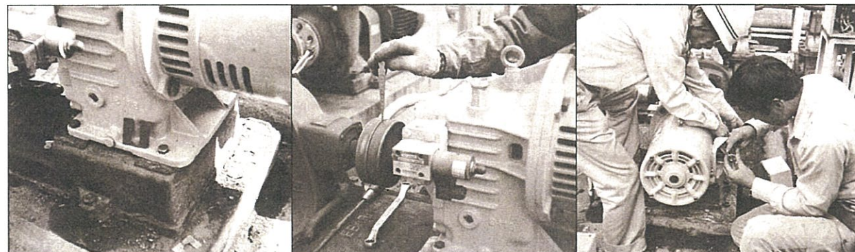
4. モータベース上にFE取付 5. カップリング芯出し 6. (制御盤取付工事後) モータ電源結線、電磁弁結線
